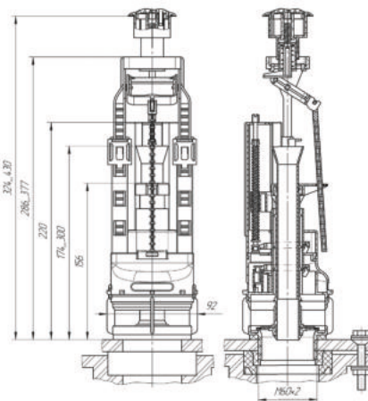
Габаритные и присоединительные размеры
